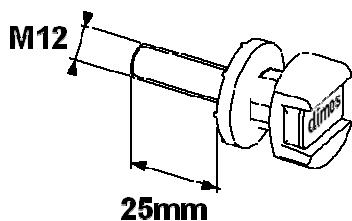
Fig. 3: ancoraggio MG3
