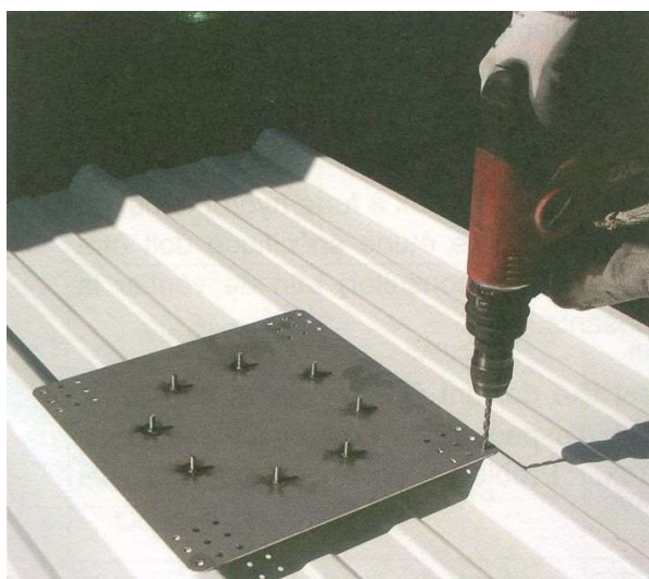
Figura 2: pre foratura da 6 mm
